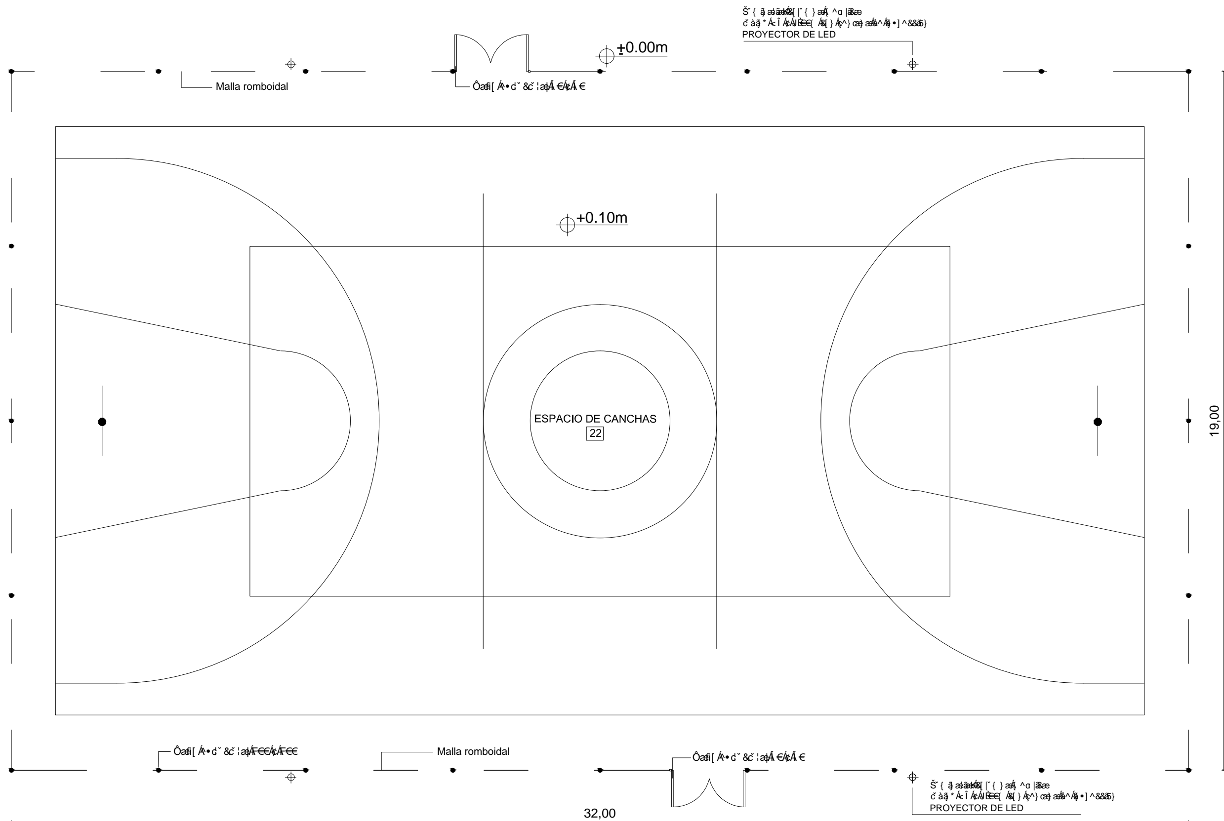
PLANTA Esc 1:100
