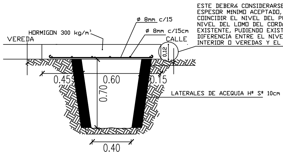
CORTE PUENTE PEATONAL
